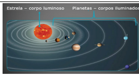
Figura 4: Corpos luminosos e corpos iluminados no S.S.
