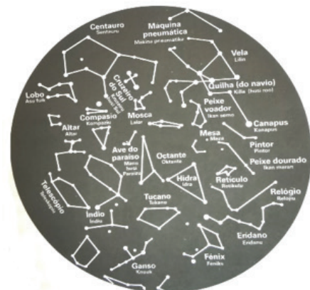
Figura 7: Constelações visíveis do Hemisfério Sul.
