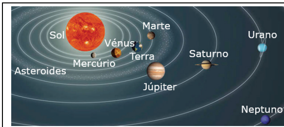
Figura 3: Sistema Solar (S.S.)
