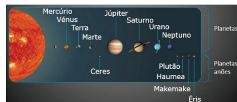
Figura 5: Constituição do Sistema Solar
